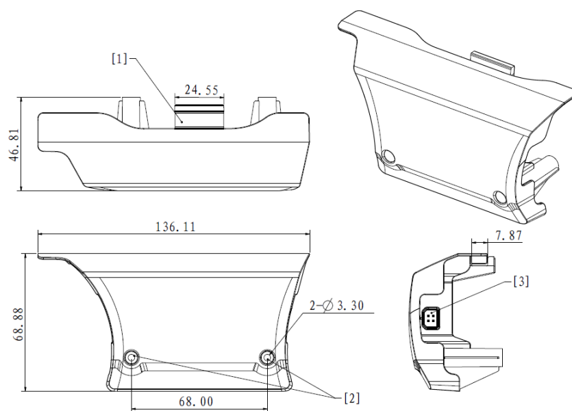
图 十-5 前装甲模块示意图
