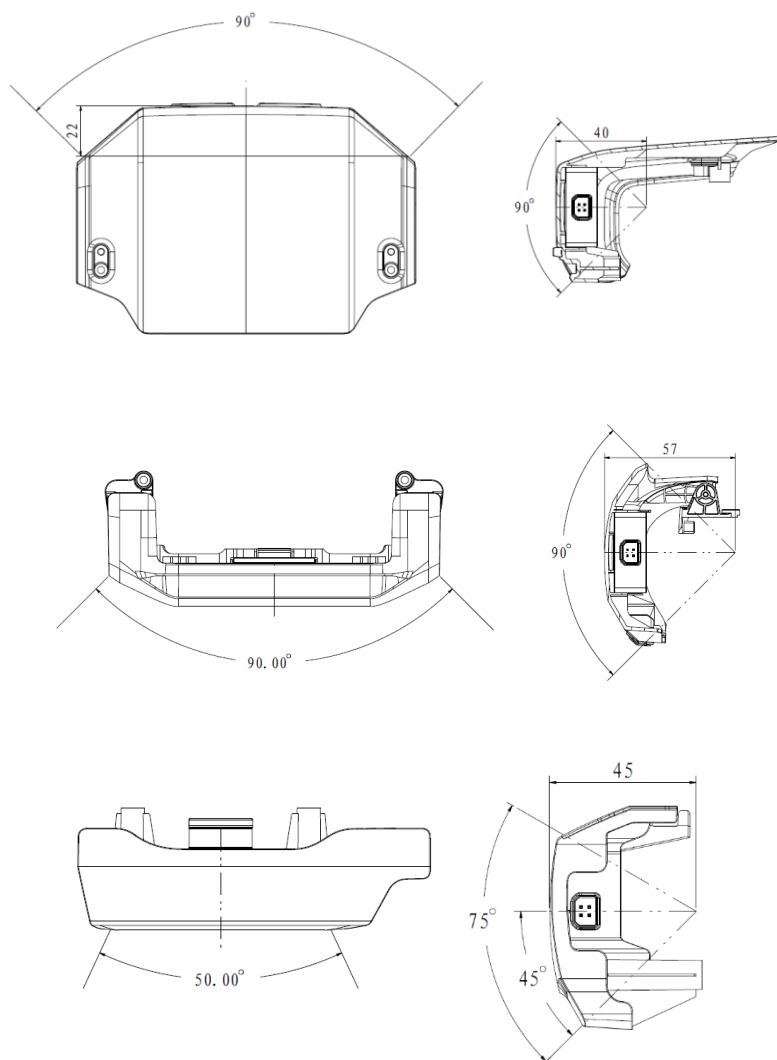
图 十-11 装甲安装规范示意图
